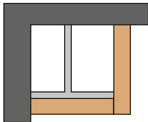
Двухсторонняя изоляция \Pi = H + S (m)
